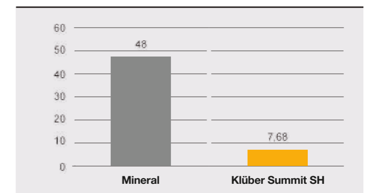
Diferencia en el contenido de vapor entre Klüber Summit SH 46 y un aceite convencional para compresores de base mineral
